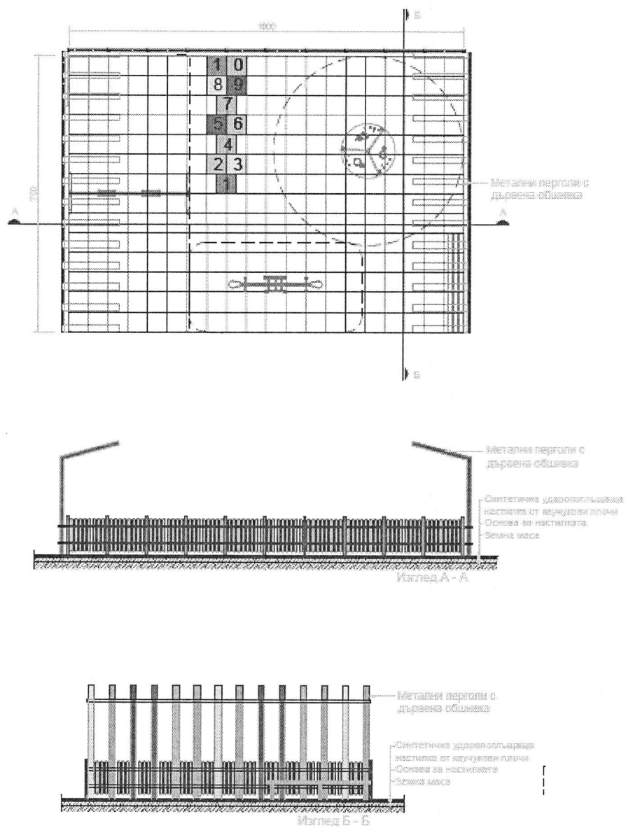
ФРАГМЕНТ НА ОГРАДА И ПЕРГОЛИ НА КЪРТ ЗА ИГРА 700/1000 cm
